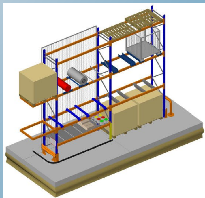
Soporte Contenedor
